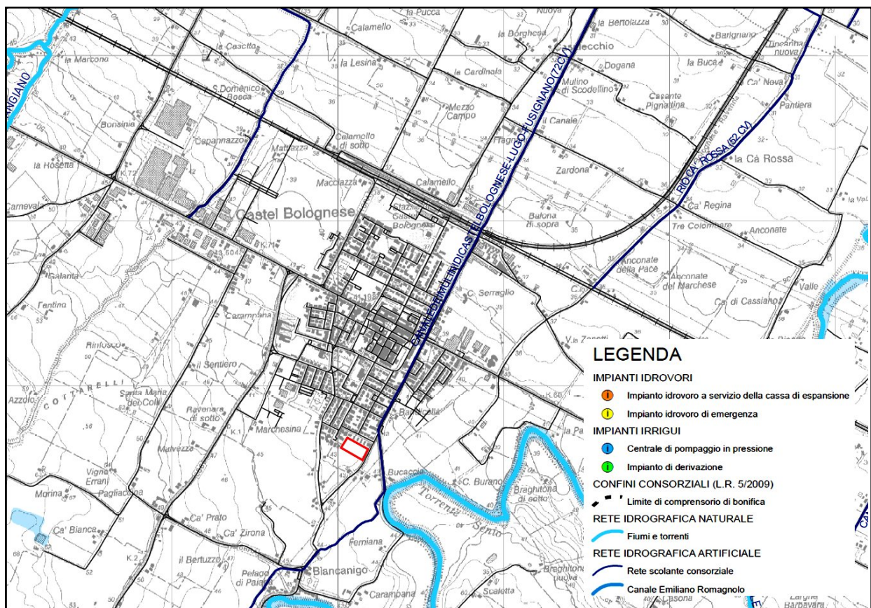
Fig. 7 - Inquadramento reticolo idraulico superficiale – rete scolante
